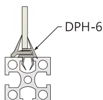
置中式壓條 側視示意圖
