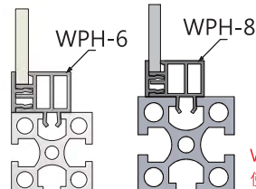
齊邊式壓條 側視示意圖
